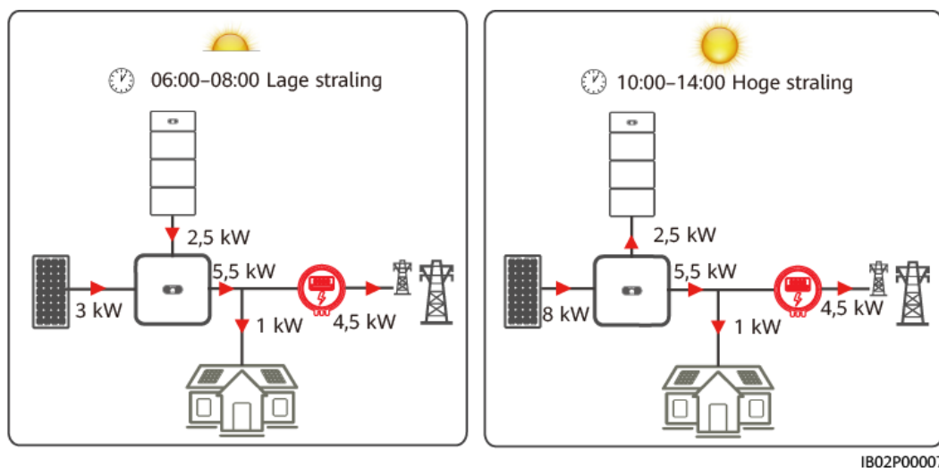
Afbeelding2-15 Volledig geleverd aan net
