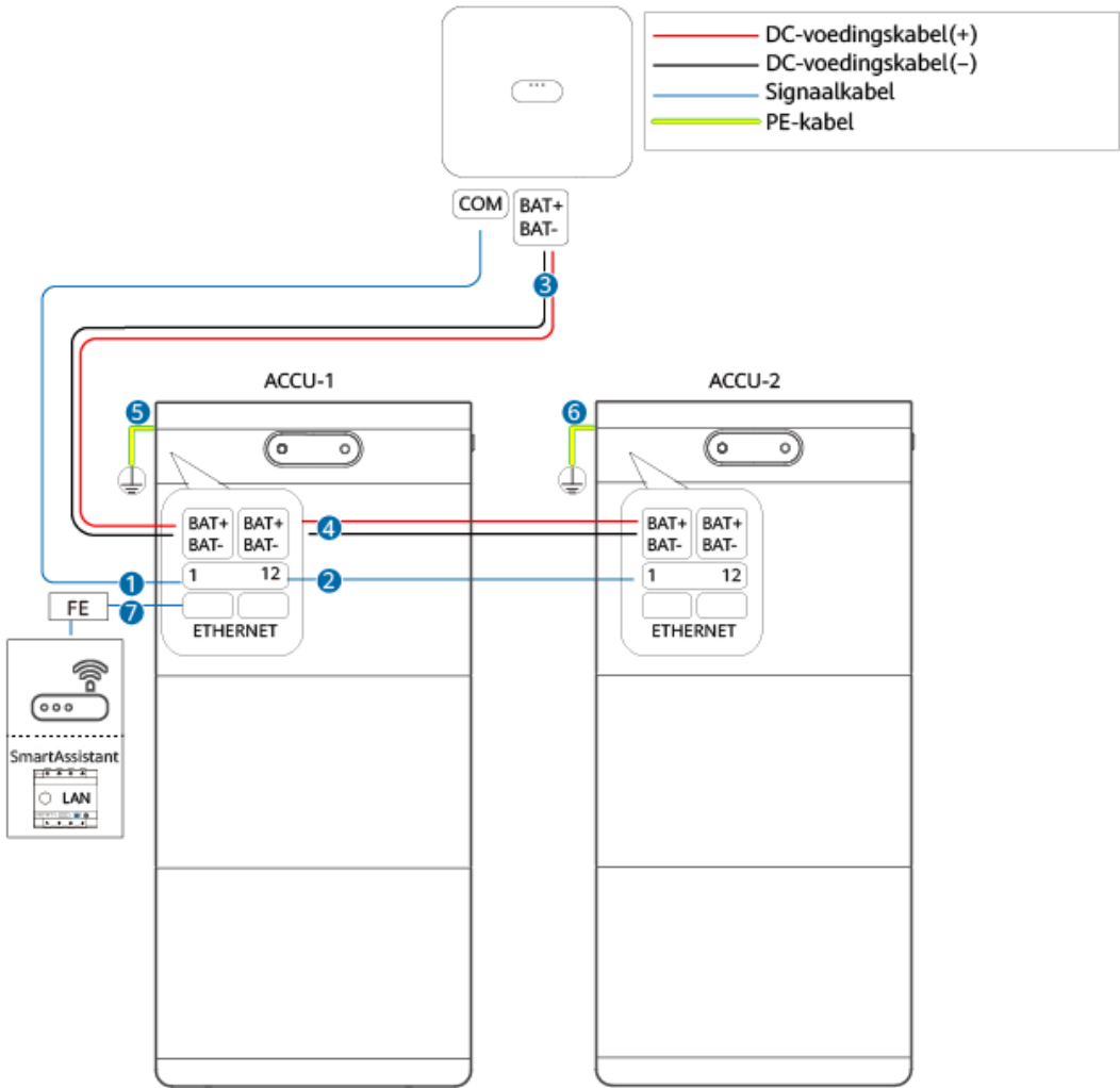
Afbeelding5-1 ESS-kabelaansluitingen
