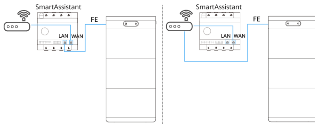
Afbeelding5-8 Netwerkpoot aangesloten op de SmartAssistant of router
