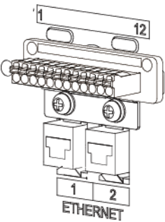
Afbeelding5-5 Signaalpoort
